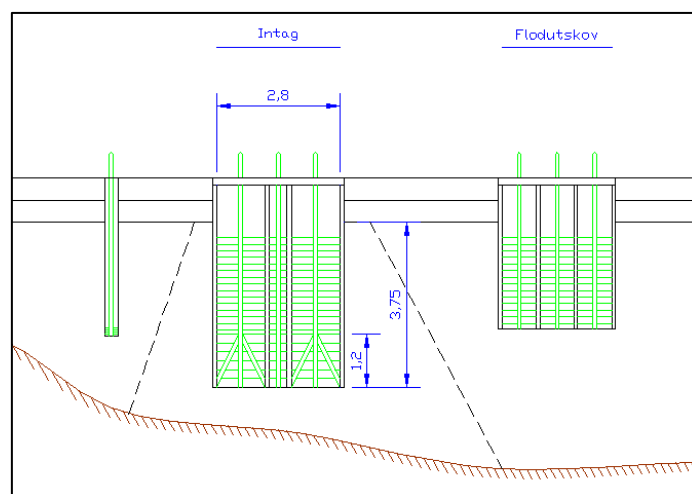
Figur 2: Medströmsvy över dambyggnaden vid intaget. Planken ovan lucköppningen fungerar som ytläns. Avståndet mellan intaget och flodutskovet är ca 3,5 m. Den smala luckan längst till vänster användes tidigare för att släppa fram vatten till en ålyngelledare.
